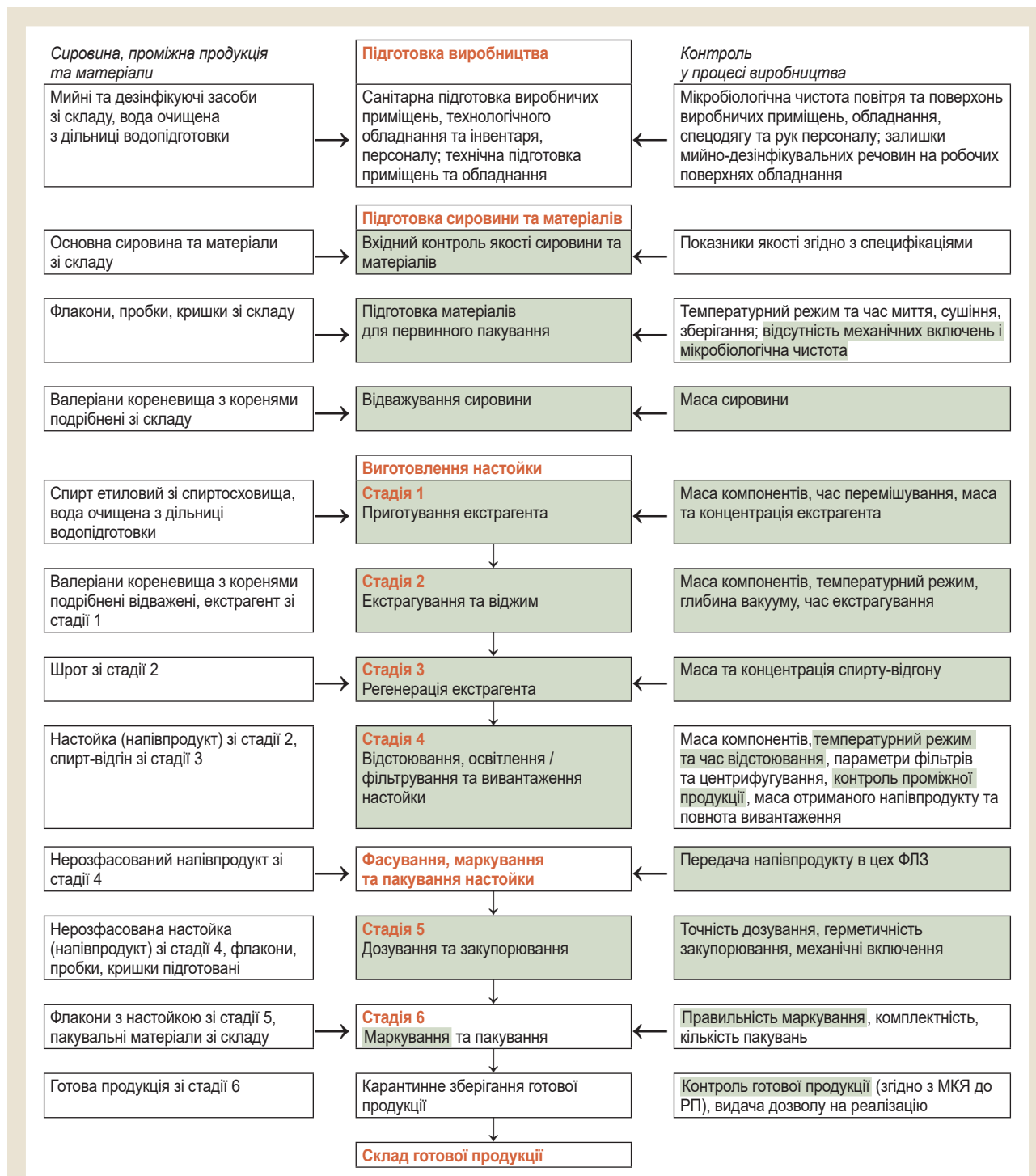
Рис. 1. Технологічна схема виробництва препарату «Валеріани настойка» по 25 мл у флаконах. *: зеленим кольором позначені критичні стадії та критичні точки контролю у процесі виробництва.
